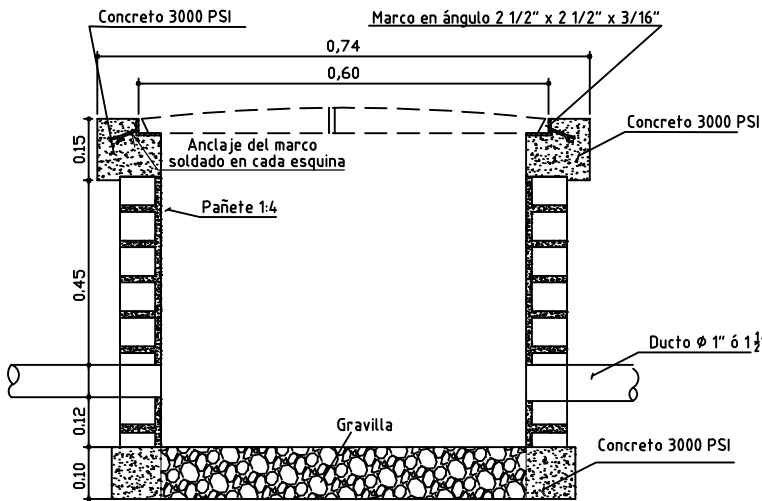
CORTE TRANSVERSAL
