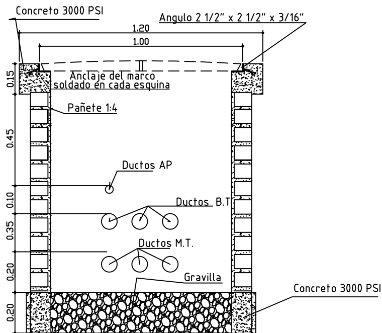
CORTE TRANSVERSAL
